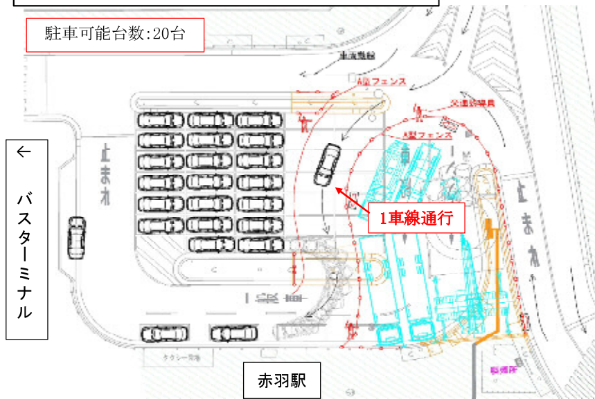
(3) ③箇所・立坑工事施工時作業帯図(21:00～(翌)6:00)
