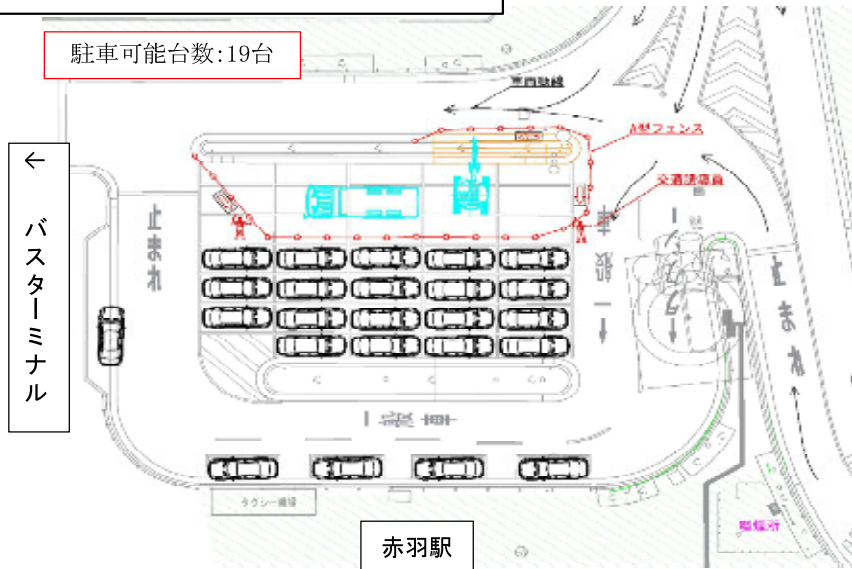
(1) ①箇所施工時作業帯図(21:00～(翌)6:00)
